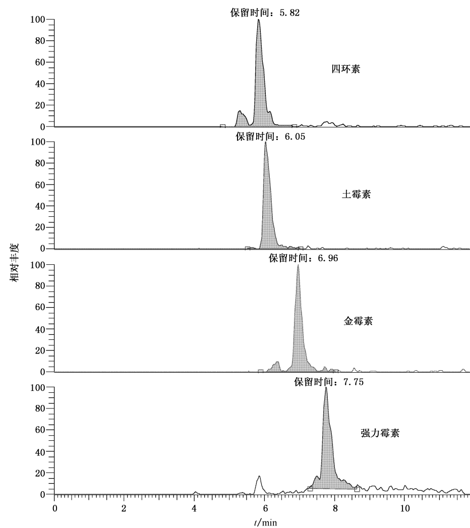
图 C.1 四环素、土霉素、金霉素、强力霉素药物标准物质分离流图
